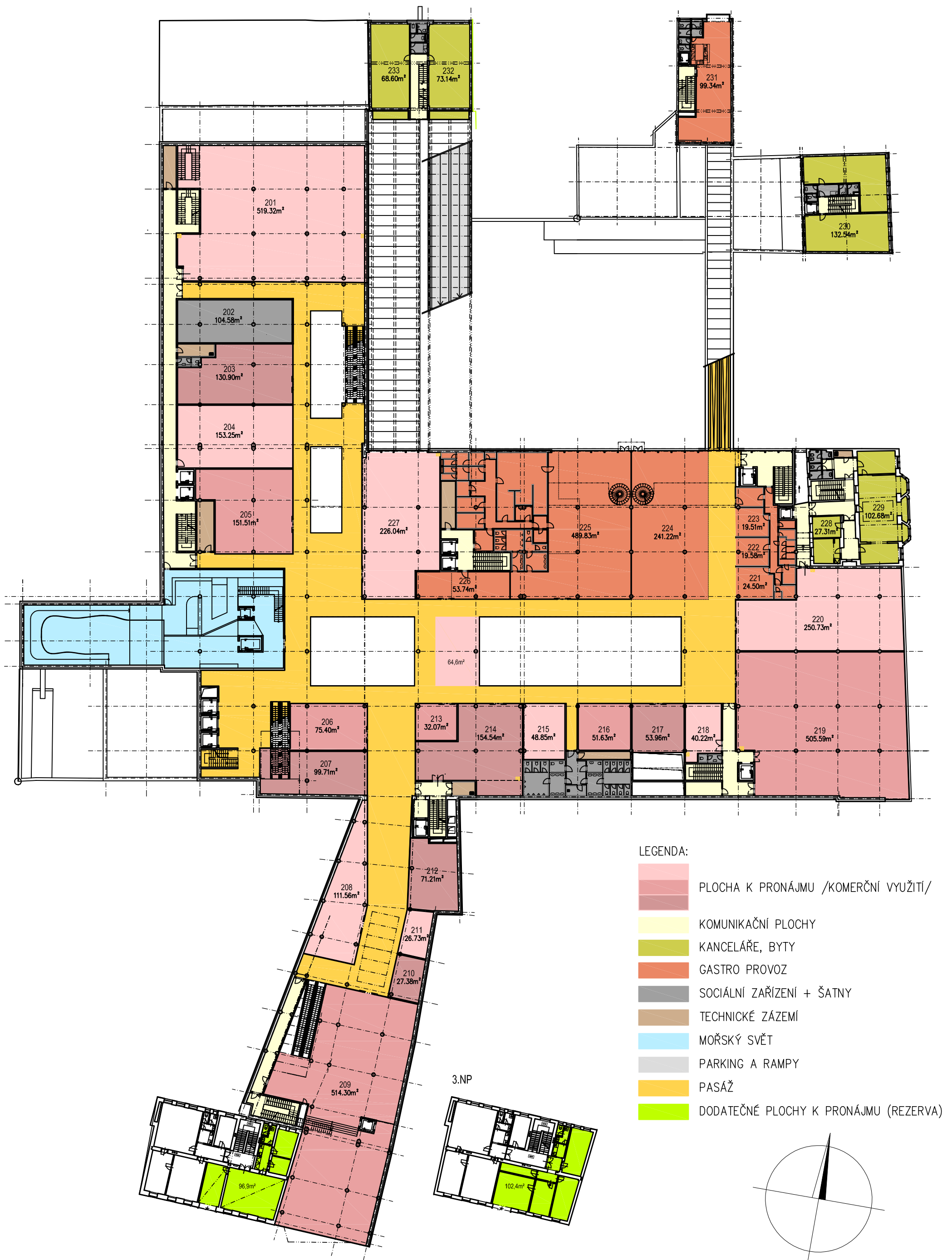
PŮDORYS 2NP 1:500
